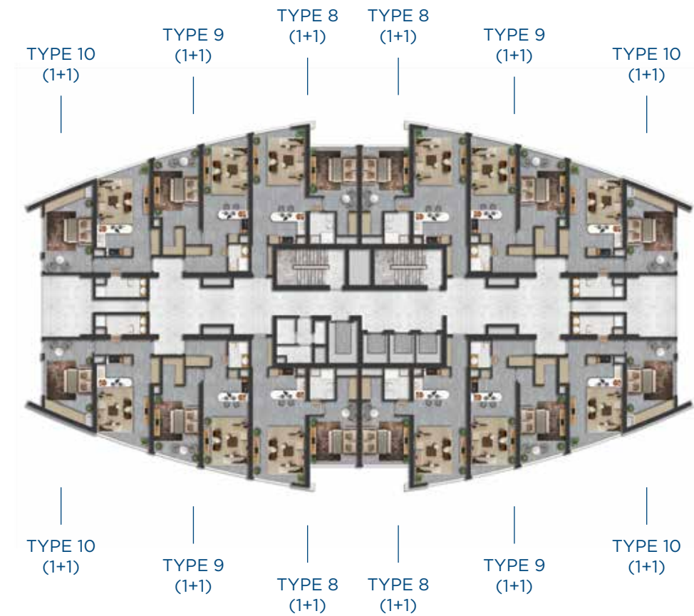
Typical Floor Type 2 مخطط طوابق النوع الثاني
