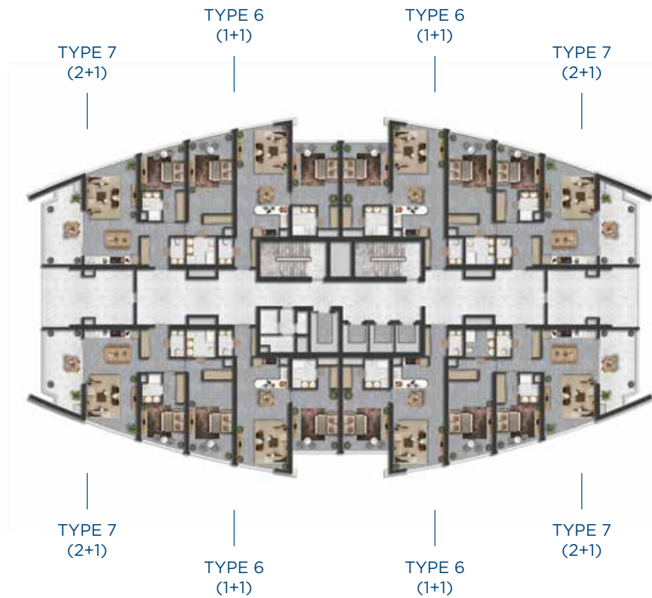
Typical Floor Type 1 مخطط طوابق النوع الأول
