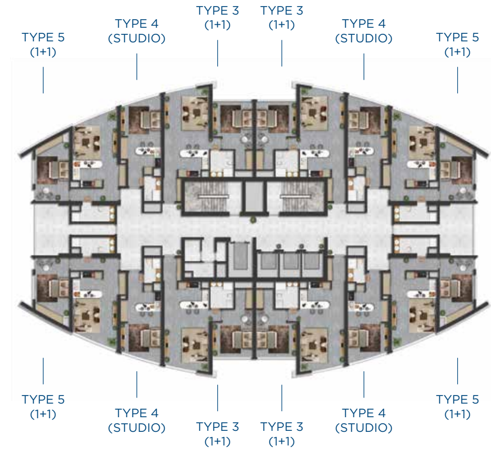
Typical Floor Type 2 مخطط طوابق النوع الثاني
